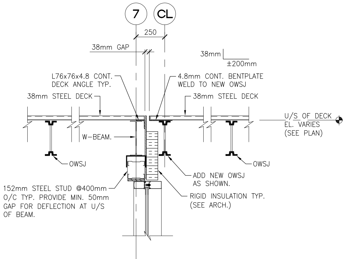
1 SECTION SR-1B SCALE: 1:20
