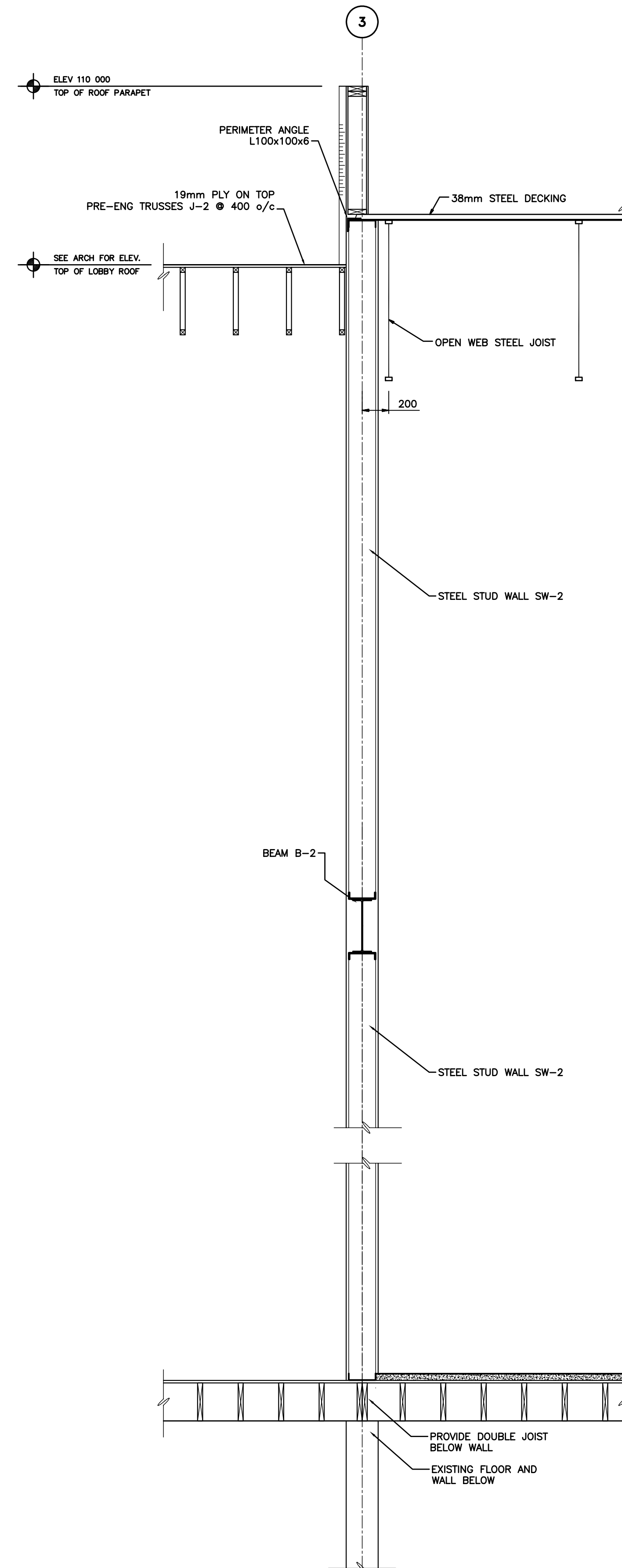
2 SECTION S-5 1 : 25
