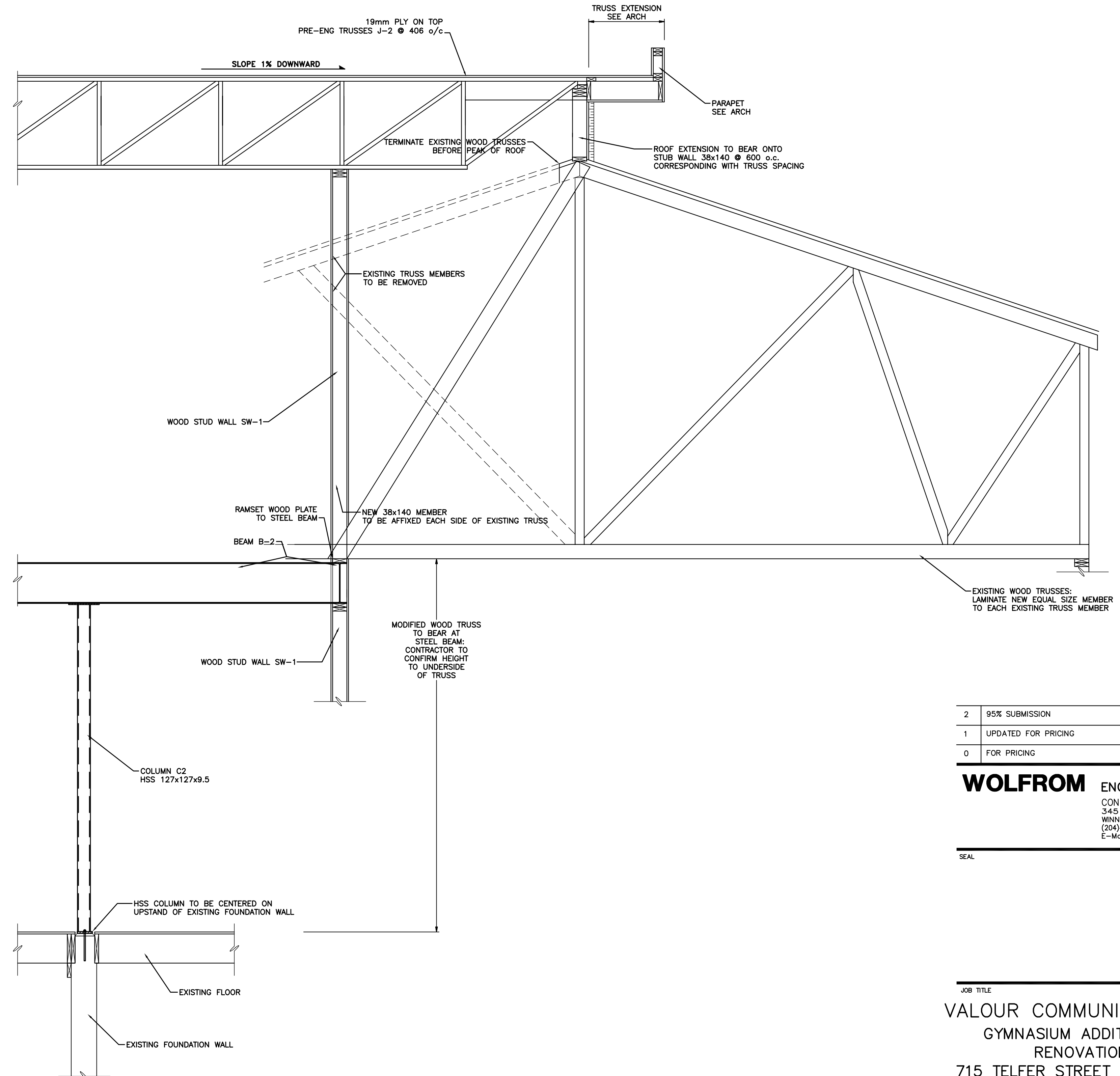
3 SECTION S-5 1 : 25
