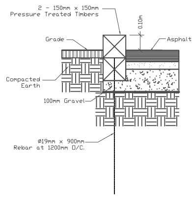
1 D2 Timber Rebar Detail
